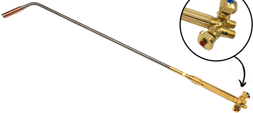
-ORCH -36"/2HC (OXY/ACY)
