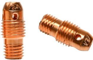
COLLET BODY -WP9
