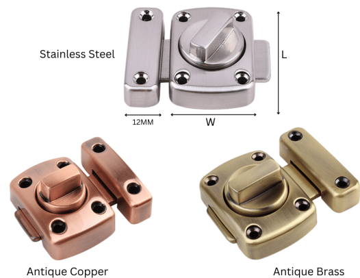
MINI DOOR LATCH (L42mm X W30mm)
