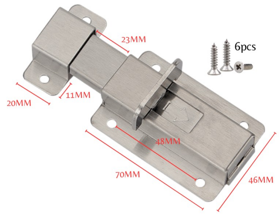
TOILET LATCH—3" | S.STEEL [4-089] SA
