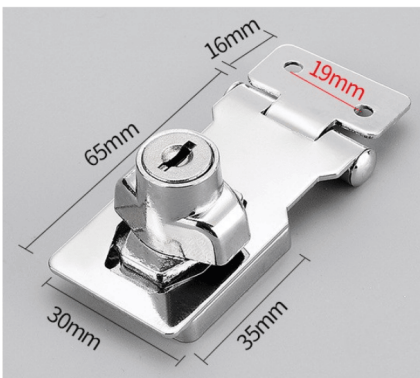
DOOR HASP LOCK - 2 1/2" [18-066] SA
