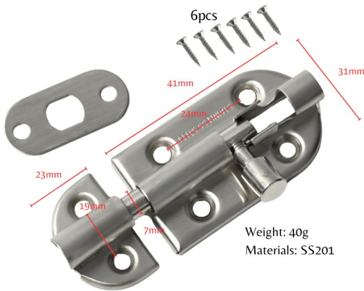
DOOR LATCH—2" | S.STEEL [4-092] SA
