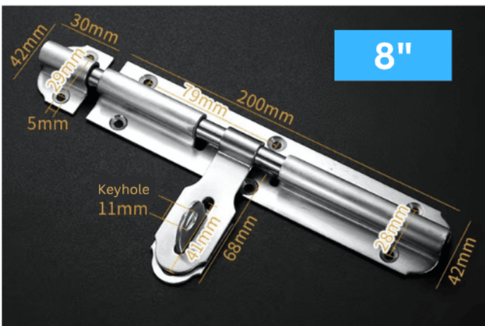
BARREL BOLT—S.STEEL / H. DUTY
