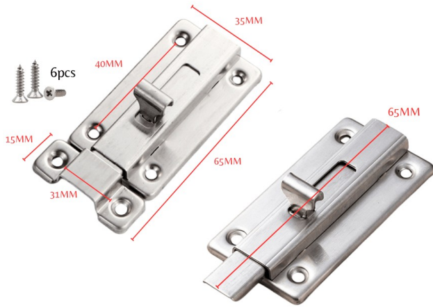
TOILET LATCH—2" | S.STEEL [4-087] SA
