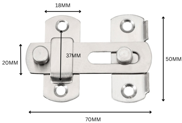
SLIDING DOOR LATCH—3" (L50MM x W70MM)
