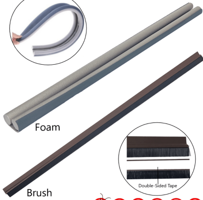
DOOR SEAL
