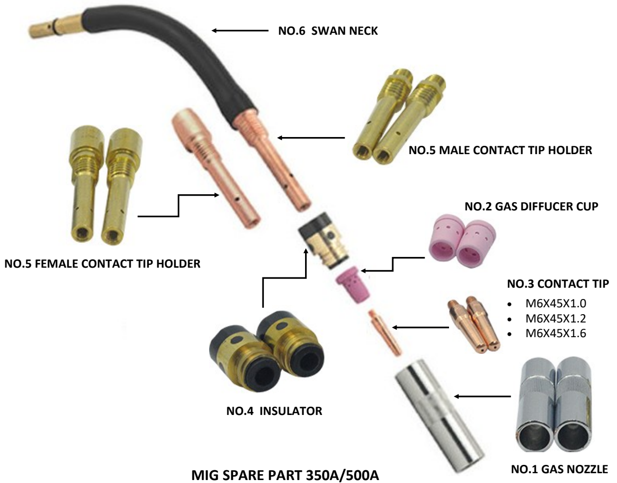
350A MIG TORCH
